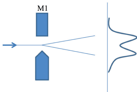
Figur 1: Principskiss över Stern-Gerlach-försöket. En stråle av partiklar med \text{spinn} = 1/2 kommer från vänster in mot en lämplig magnet, M1, där strålen splittras upp beroende på om spinnet är upp eller ned. Fördelningen av partiklarna på skärmen till höger visar denna uppdelning.
