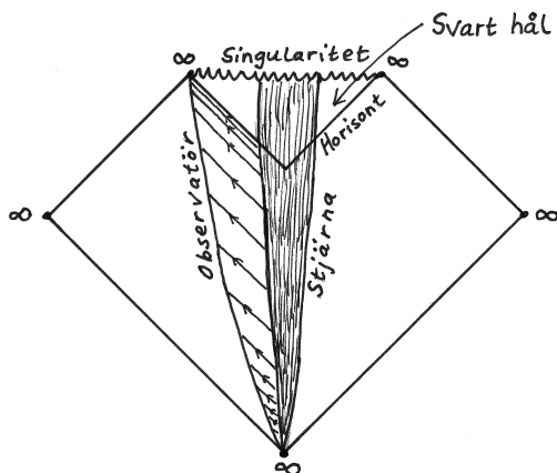
Figur 9: Ett annat sätt att se på sfäriskt symmetrisk gravitationskollaps. Istället för den lätt impressionistiska Figur 8 ritar vi ett konformt Penrose-diagram, där avstånden är förryckta men ljussignaler alltid utväxlas längs linjer som lutar 45 grader. Speciellt lutar händelsehorisonten i 45 graders vinkel. Vi ser nu tydligt att singulariteten inte ligger i centrum av stjärnan, den ligger i (eller avslutar) dess framtid. Det svarta hålet består av den del av rumtiden från vilken inga signaler kan nå oändligheten. Observatören befinner sig utanför det svarta hålet och rör sig längs en världslinje som går från förfluten oändlighet till framtida oändlighet. Signaler som skickas från punkter inne i det svarta hålet kommer att träffa singulariteten, och når aldrig observatören.
