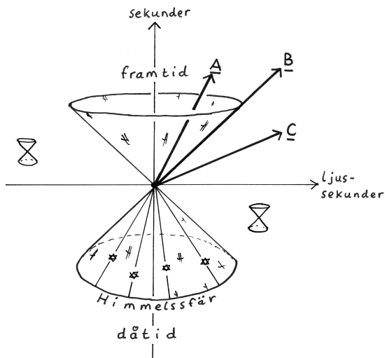
Figur 2: En karta över en del av Minkowskis rumtid. Enheterna har valts så att ljushastigheten c = 1 ljussekund/sekund. Varje punkt ligger i spetsen på en dubbelkon som kallas ljuskonen. Om vi kunde rita en fyrdimensionell bild skulle vi se att konens bas är en två dimensionell sfär som vi här kallar himmelssfären. Från varje punkt leder tre olika slags riktningar, tidsartade (A), ljusartade (B), och rumsartade (C). De ljusartade riktningarna ligger på ljuskonen. De tidsartade leder in i konen, och de rumsartade ut ur den. Rör man sig i en ljusartad riktning färdas man med ljusets hastighet. Ingenting kan färdas i en rumsartad riktning eftersom ingenting kan färdas snabbare än ljuset. Från en given punkt kan man bara se de händelser som utspelar sig på den bakåtriktade ljuskonen.
