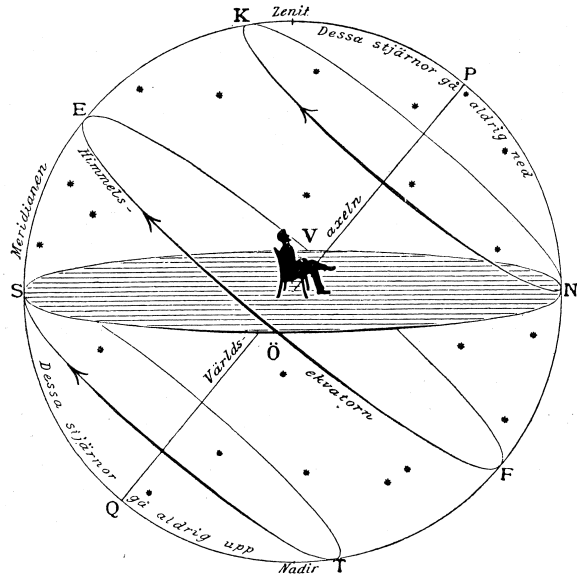
Figur 4: Himmelssfären. från C. Rendahl och B. Söderborg, Astronomi , Norstedt & Söner 1931.
