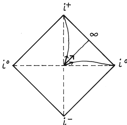
Figur 7: Ett Penrosediagram för det två dimensionella Minkowskirummet, jämför Figur 2. Går vi från origo oändligt långt längs en rumsartad riktning hamnar vi i en oändlighetspunkt som kallas i^o . Går vi oändligt långt i en tidsartad riktning hamnar vi i framtida oändlighet i^+ . Diagrammet är ritat så att ljusartade riktningar alltid lutar i 45 graders vinkel. Följer vi en ljussignal till oändligheten hamnar vi i en tredje sorts oändlighet, som bildar diagrammets rand (här markerad med " \infty ").
