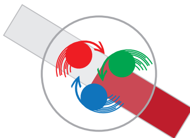
Figur 1: Protonens magnetiska moment uppstår tack vare rörelsen hos dess laddade beståndsdelar.
