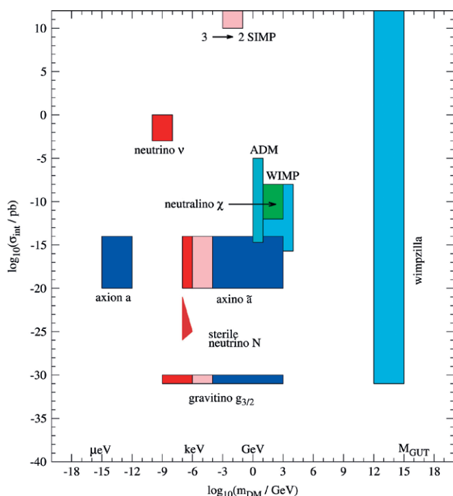
Figur 4: Några utvalda modeller för mörk materia, åskådliggjorda i ett plan med mörk materie-massan på den horisontella axeln och växelverkanstyrkan (”tvärsnittet”) på den vertikala. Notera att båda axlarna täcker in ett brett intervall av olika storleksordningar. Se vidare sidorutan. (Figur från H. Baer, K. Y. Choi, J. E. Kim och L. Roszkowski, Phys. Rep. 555 , 1 (2015) (DOI: 10.1016/j.physrep.2014.10.002). Återpublicerad med tillstånd från författarna.)
