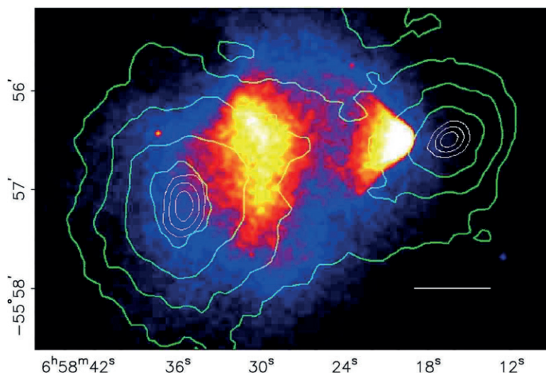
Figur 3: Gevärskulehopen avbildad på två olika sätt. Ljusa partier motsvarar områden med hög intensitet utsänd röntgenstrålning, och därmed områden med hög täthet av vanlig (ljusutsändande) materia. Effekter från gravitationslinsning av ljus från bakomliggande galaxer är markerade med gröna nivåkurvor: linsningseffekterna är små längs de yttre nivåkurvorna, och större längs de inre. Detta ger en bild av hur den totala massan är fördelad i systemet. Skillnaden mellan de två fördelningarna kan bara förklaras av att kollisionen mellan galaxhoparna även innefattade en andel mörk materia. (Bild från D. Clowe et al., Astrophys. J. 648 , L109-L113 (2006) (DOI: 10.1086/508162). Återpublicerad med tillstånd från författarna.)
