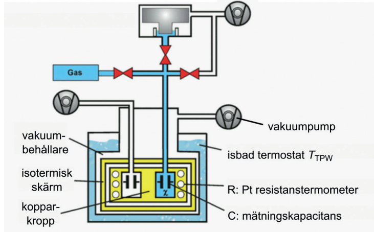
Figur 8. Schematisk bild av den kapacitiva mätinrättningen [6] för heliums dielektriska susceptibilitet \epsilon_r - 1 . Referenskondensatorn i vakuum ligger till vänster och mät-kondensatorn fylld med He-gas vid tryck p till höger. Kondensatorerna är inbäddade i en termostat vid konstant temperatur T_{TPW} , som observeras med flera platina resistanstermometrar. Alla dessa delar ligger inom en vakuumbehållare. Tryckmätningen sker med en klassisk mekanisk balansvåg. Bild: © Bureau International des Poids et Mesures and IOP Publishing Ltd. Reproduced by permission of IOP Publishing. All rights reserved.
