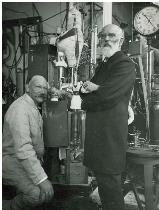
Figur 2. Professorerna Kamerlingh Onnes och Johannes van der Waals i lågtemperaturlaboratoriet vid Leiden universitetet. Året är 1913 när Kamerlingh Onnes belönades med Nobelpriset för sina forskningar vid låga temperaturer som hade lett till kondensation av helium. Kollegan van der Waals hade fått sitt Nobelpris 1910 för utvecklingen av tillståndsekvationen för gaser och fluider.
