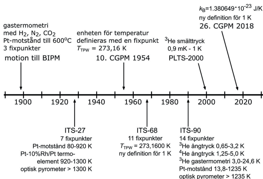
Figur. 3. Tidslinjen för de viktigaste åtgärderna för att fixera den internationella temperaturskalan ITS som överses av Conférence Générale des Poids et Mesures (CGPM). Skalan är baserad på internationella överenskommelser om vilka fixpunkter som ska användas för kalibrering och deras värden, samt mätningsteknikerna och analytiska formuleringar för en slät och kontinuerlig interpolation av mätvärdet som funktion av temperaturen.
