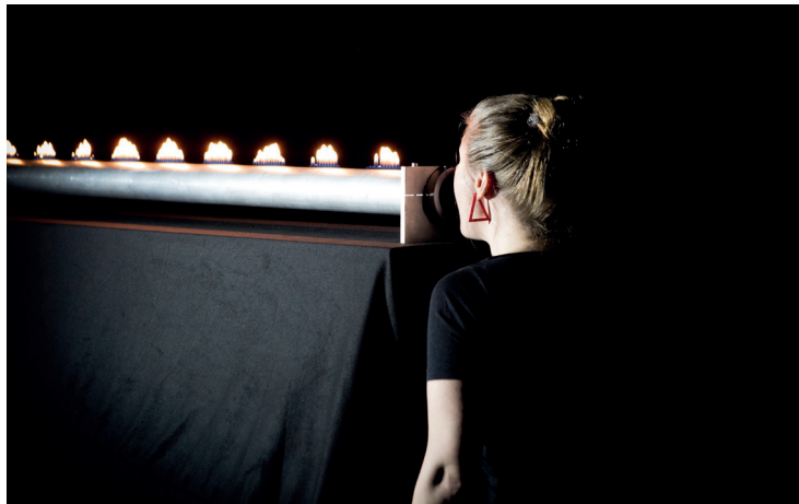
Figur 3: På bilden ser ni hur det skapas en stående våg i röret när Hedvig Jalhed tar en ren ton. Vid tryckbukarna kommer flammorna att vara högre och vid noderna trycks det inte ut någon gas alls. För en stående våg är avståndet mellan två bukar en halv våglängd. För att skapa en stående våg i röret måste randvillkoren vara uppfyllda, så det är bara vissa frekvenser som skapar fenomenet. Om man sjunger i röret kommer flammorna därför att hoppa runt. I filmen som ni kommer till via QR-koden (se efter ”Vidare läsning”) sjunger Hedvig en bit ur arian Lascia ch’io pianga av Händel (foto: Magnus Pålsson).
