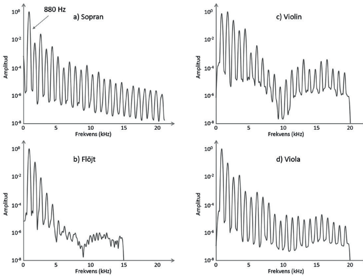
Figur 6: Frekvensanalys av ljudet från en sopran som sjunger tvåstrukna A och samma ton för tre olika instrument: a) Hedvig Jalhed sjunger tvåstrukna A (880 Hz), b) tvåstrukna A på en tvärflöjt, c) violin och d) viola. Övertoner från sopranen täcker hela det hörbara området och avtar inte lika fort som till exempel flöjten. Violin och viola är instrument med mycket rika övertonsspektra. Även om de påminner mycket om varandra går det att se en tydlig skillnad i frekvensstrukturen när de tar samma ton.
