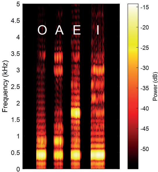
Figur 8: Frekvensanalys av fyra olika vokalljud sjugna med samma grundton. Alla vokalerna har 440 Hz som grundton, men strukturen på övertonerna med olika formanter gör att vi hör dem som olika vokalljud.
