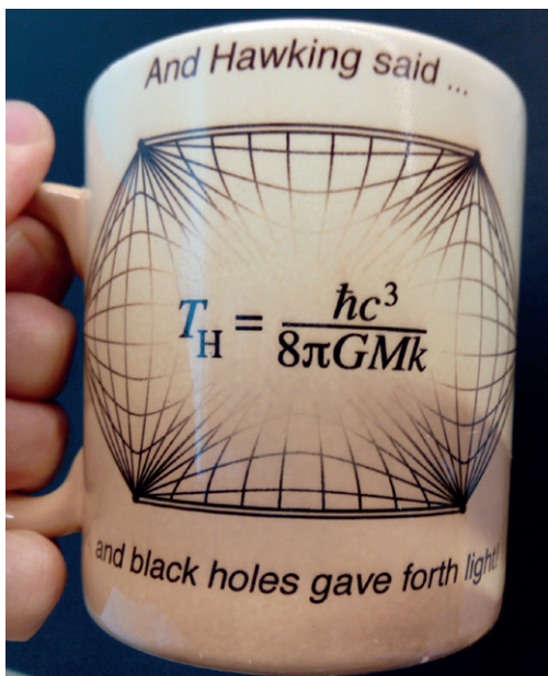
Figur 1: Jag var på Hawking's 60-årskalas och fick den här fina kaffekoppen. Den var helsvart tills man hällde i varmt kaffe, då trädde formeln fram. Tyvärr rådde den hamna i diskmaskinen, så nu är den alltid vit.
