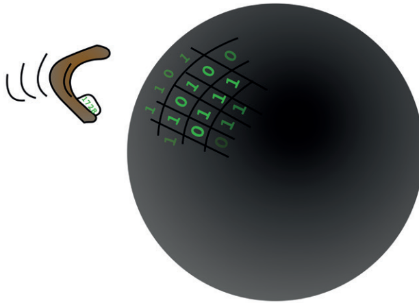
Figur 2: Brian Greene kastar in sin plånbok i ett svart hål. Sfäriskt symmetriska svarta hål karaktäriseras enbart av sin massa M . Så vad händer med informationen som finns lagrad i bankkortschipet?
